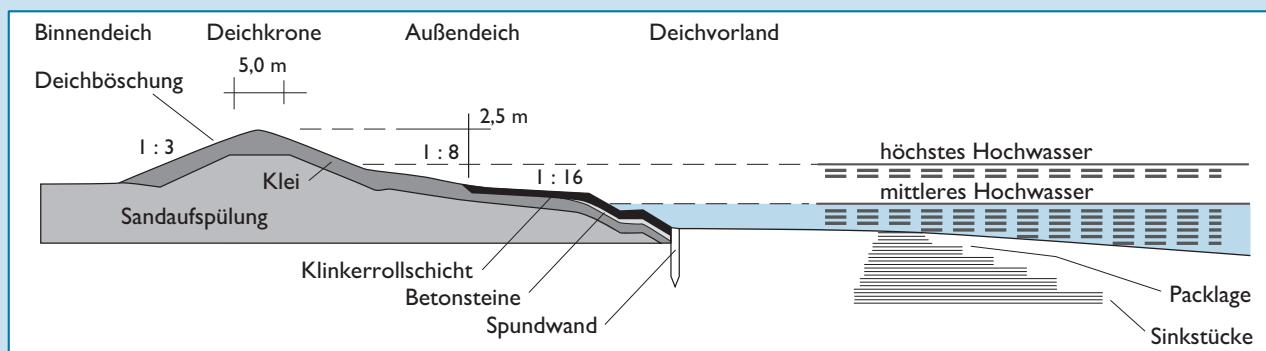
Querschnitt eines Deichs
