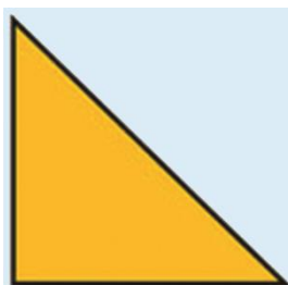
चित्र 2 समकोण त्रिभुज।
