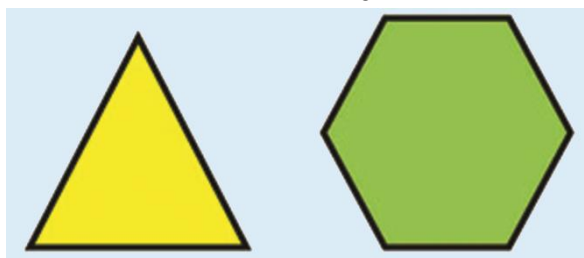
चित्र 1 एक समबाहु त्रिभुज और षट्कोण।
