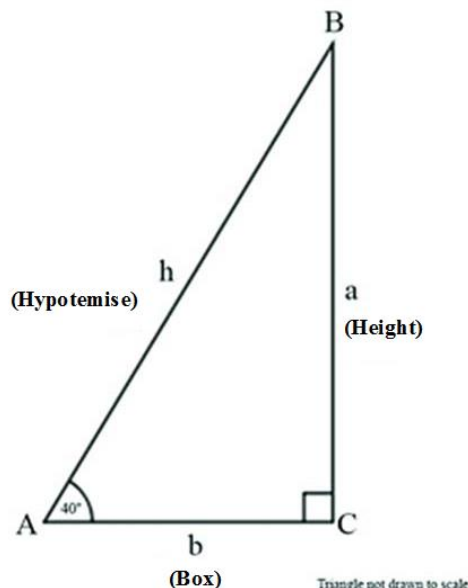
चित्र 4 समकोण त्रिभुज का एक उदाहरण।
