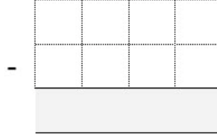
चित्र 4 एक व्यवकलन ग्रिड।
